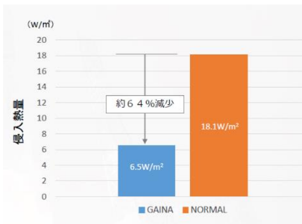
侵入熱量を比較したグラフ
